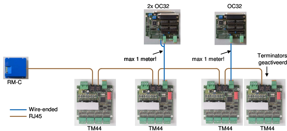
Fig 15: Eén netwerk met de RM/C als eindpunt
