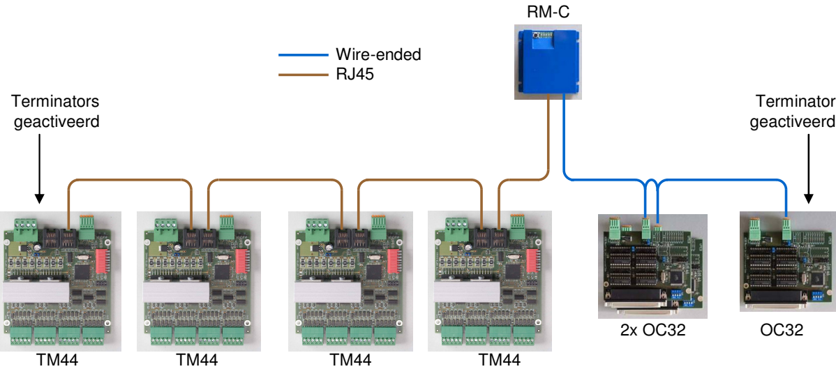
Fig 17: Eén netwerk met de RM-C als RJ45 naar wire-end tussenstation
