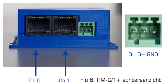
Fig 6: RM-C/1+ achteraanzicht
