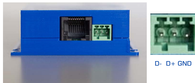
Fig 5: RM-C/1 achteraanzicht
