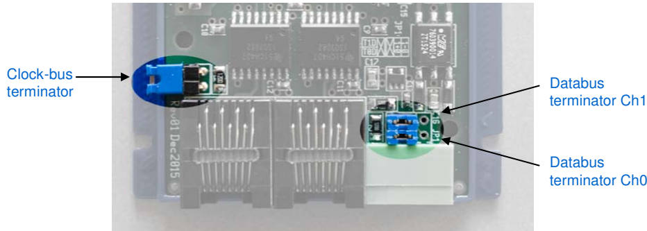
Fig 11: Jumper instellingen bij de RM-C/2
