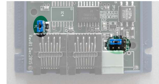
Fig 7: Jumpersettings voor RM-C/1+ als eindpunt
