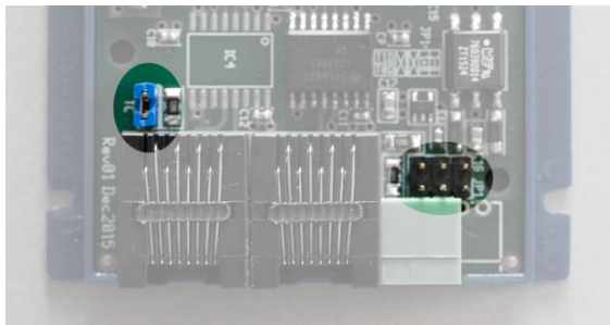
Fig 9: Jumpersettings voor RM-C/1+ als RJ45↔wire-end tussenstation
