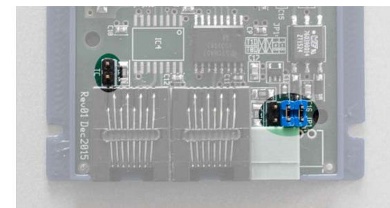
Fig 8: Jumpersettings voor RM-C/1+ als RJ45↔RJ45 tussenstation
