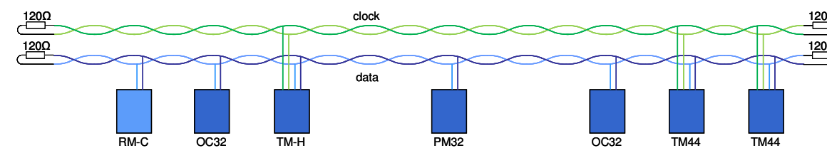
Fig 14: Clock en Databus tussen Dinamo modules
