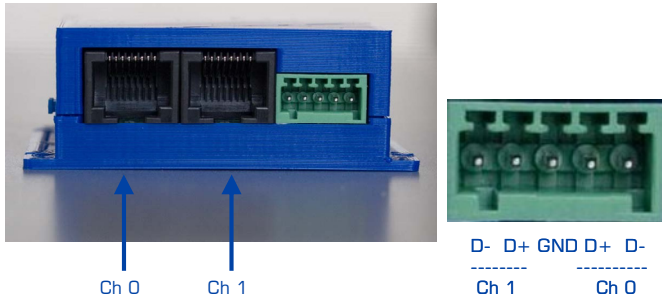
Fig 10: RM-C/2 achteraanzicht
